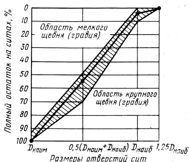
Рисунок 7.1 – Кривая отсева
