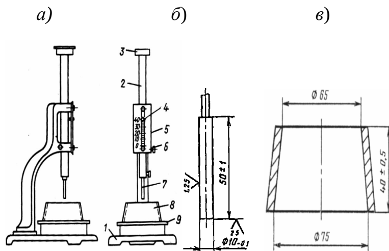
Рисунок 5.5 – Оборудование для определение нормальной густоты цементного теста
