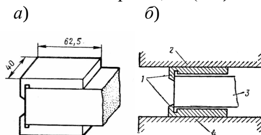
Рисунок 5.15 – Определение предела прочности при сжатии
