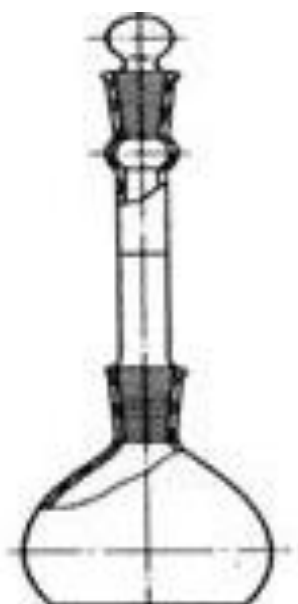
Рисунок 1.1 – Объёмомер Ле-Шателье
