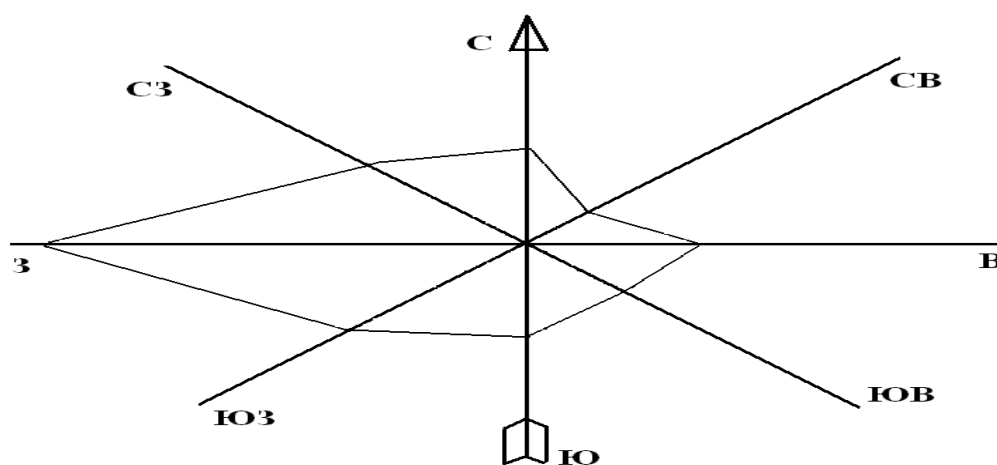
Рис. 2. Роза ветров
