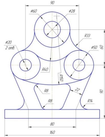
Рисунок 2 Вариант 2 Подвеска
