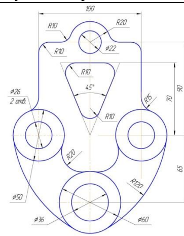
Рисунок 4 Вариант 4 Подвеска
