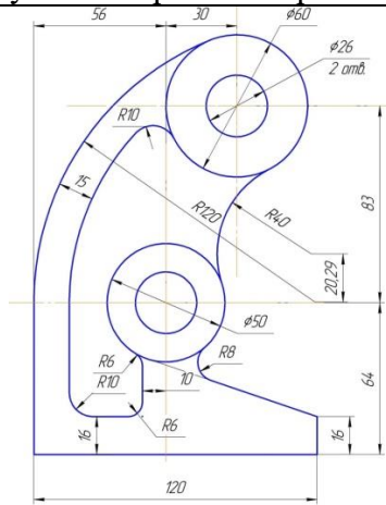
Рисунок 3 Вариант 3 Станина
