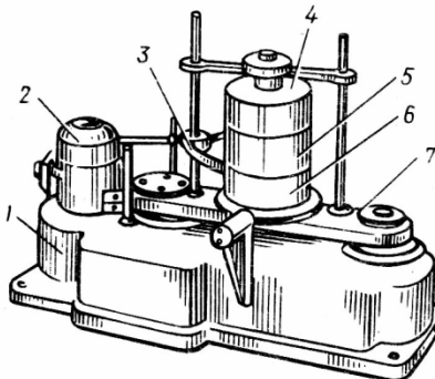
Рисунок 5.3 – Сито механическое
