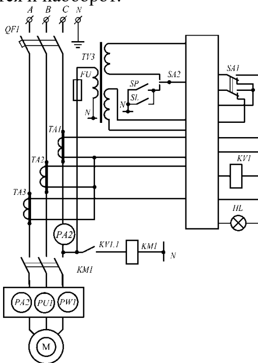
Рисунок 2 - Схема лабораторной установки
