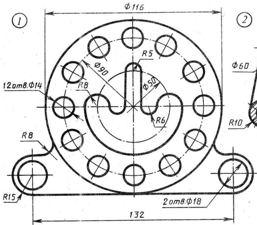
Крышка
