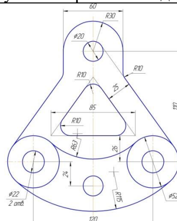
Рисунок 6 Вариант 6 Подвеска
