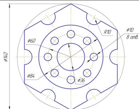
Рисунок 5 Вариант 5 Прокладка
