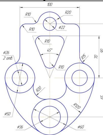
Рисунок 2 Вариант 2 Подвеска
