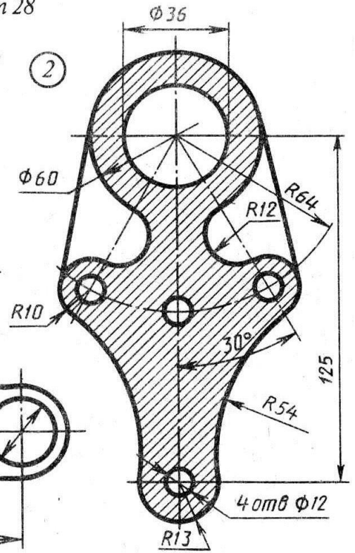
Подвеска
