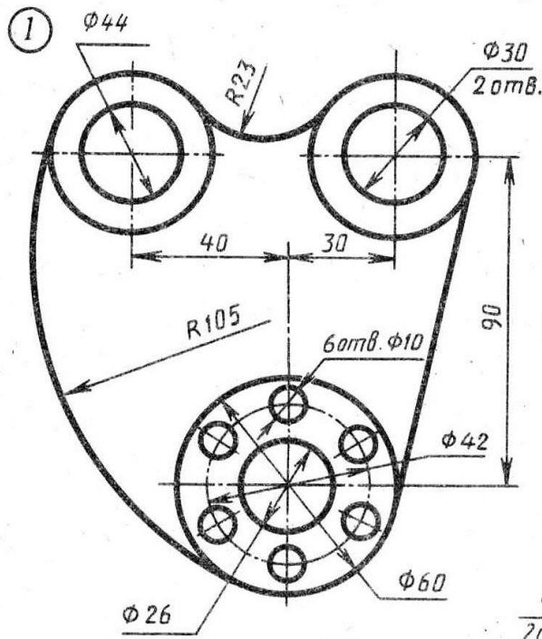
Ушко
