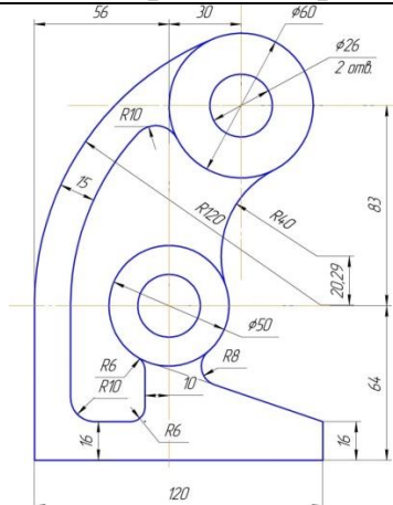
Рисунок 1 Вариант 1 Кронштейн
