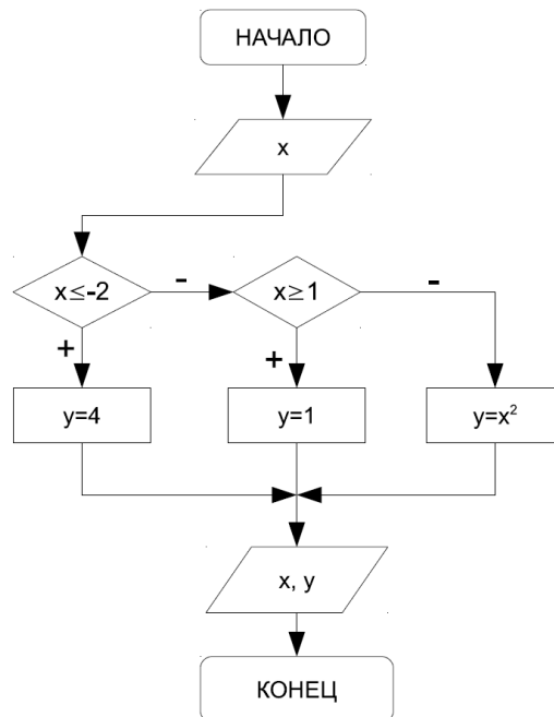
Рисунок 2- Блок-схема примерного алгоритма решения задачи
