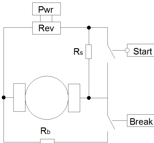
Рисунок 1 - Схема реверсивного электропривода двигателя постоянного тока без обратной связи с управлением разгоном и торможением по времени.
