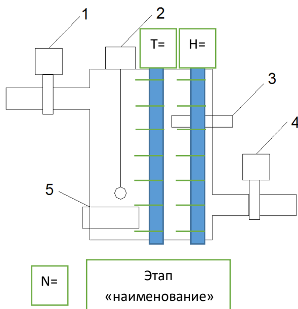
Рисунок 1 – Структурная схема установки
