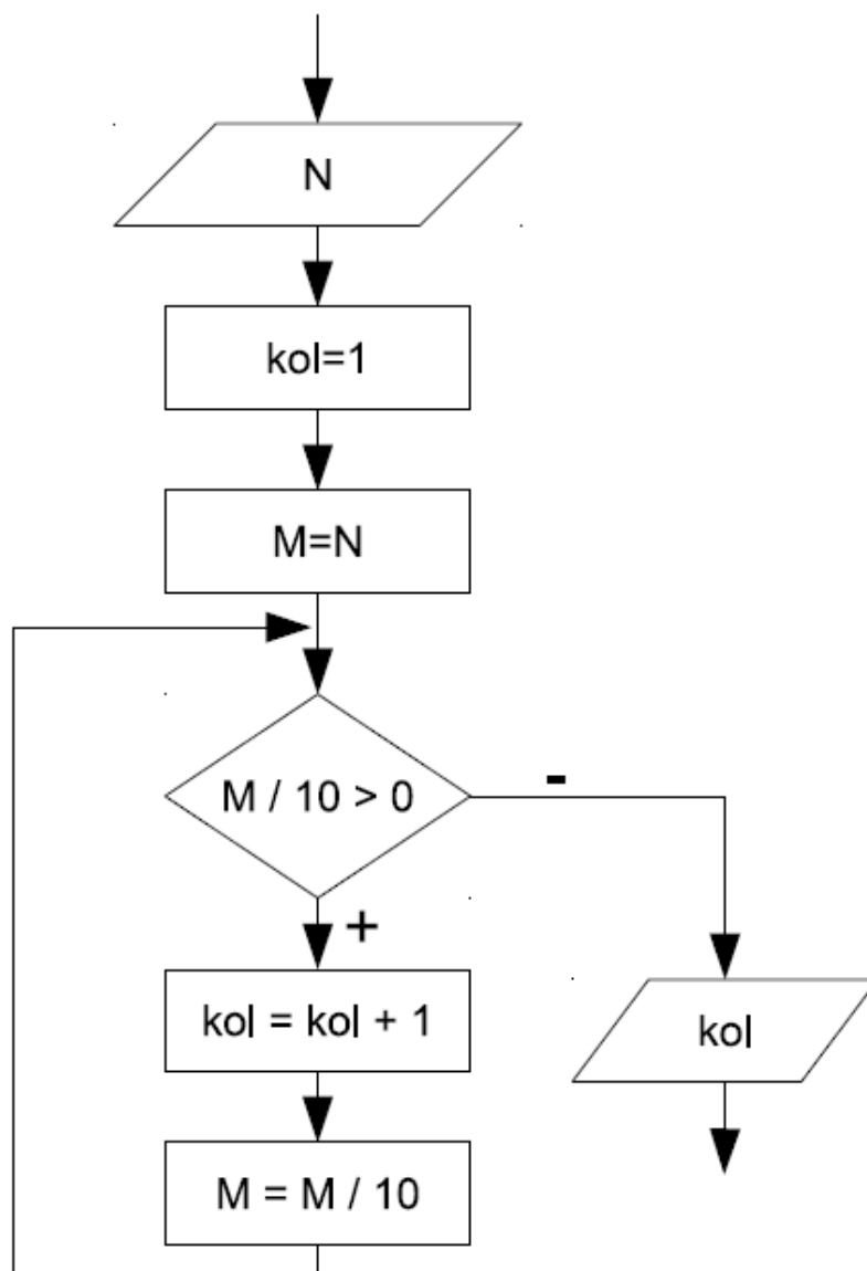
Рисунок 1 – Алгоритм вычисления
