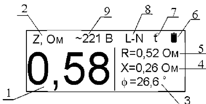
Рисунок 8.3 – Вид индикатора в режиме «фаза-нуль»: 1 – значение основного параметра; 2 – обозначение и размерность основного параметра; 3, 4, 5 – обозначение, значение и размерность второстепенных параметров; 6 – символ, индицирующий состояние батареи; 7 – символ, сигнализирующий о перегреве прибора; 8 – символ режима работы прибора; 9 – текущее напряжение в измеряемой цепи.
