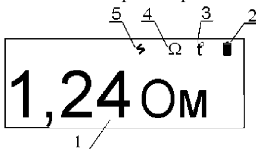
Рисунок 8.4 – Вид индикатора в режиме «Омметр»: 1 – измеренное значение; 2 – символ, индицирующий состояние батареи; 3 – символ, сигнализирующий о перегреве прибора; 4 – символ режима работы прибора; 5 – символ, сигнализирующий о присутствии напряжения на гнездах прибора.
