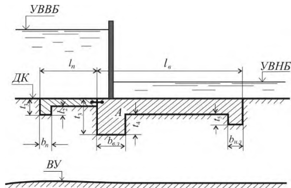
Рисунок 1 - Сечение флютбета
