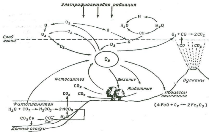
Рис. 1. Круговорот кислорода
