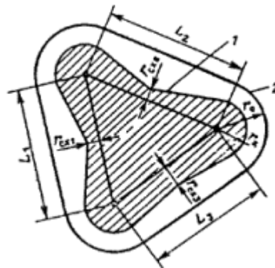
Рисунок 6 - Зона защиты (в плане) многократного стержневого молниеотвода. Обозначения те же, что и на рис. 3
