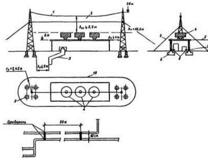
Рисунок 9 - Молниезащита здания I категории отдельно стоящим тросовым молниеотводом ( \rho = 300 \text{ Ом м} , S_0 \leq 4 \text{ м} , S_3 \leq 6 \text{ м} , S_{01} \geq 3,5 \text{ м} ):
