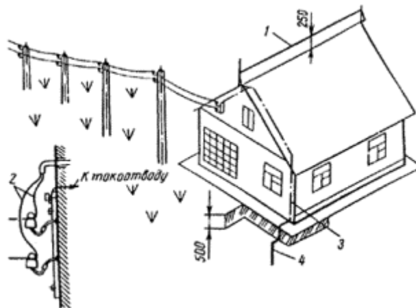
Рисунок 12 - Молниезащита сельского дома тросовым молниеотводом, установленным на крыше: 1 - тросовый молниеприемник; 2 - ввод воздушной линии электропередачи (ВЛ) и заземление крюков ВЛ на стене; 3 - токоотвод; 4 - заземлитель
