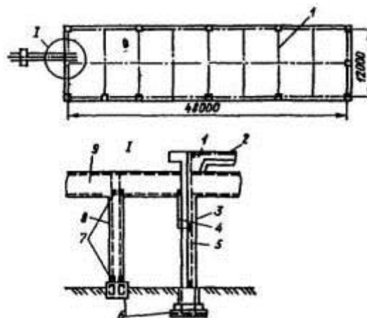
Рисунок 10 - Молниезащита здания II категории сеткой, уложенной на кровлю под изоляцией: 1 - молниеприемная сетка; 2 - гидроизоляция здания; 3 - опора здания; 4 - стальная перемычка; 5 - арматура колонны; 6 - заземлители - железобетонные фундаменты; 7 - закладная деталь; 8 - опора эстакады; 9 - технологическая эстакада
