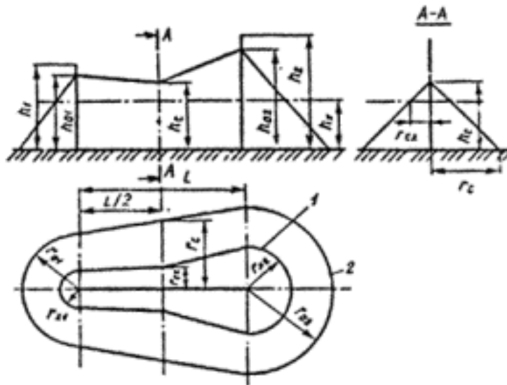
Рисунок 5 - Зона защиты двух стержневых молниеотводов разной высоты. Обозначения те же, что и на рис. 3
