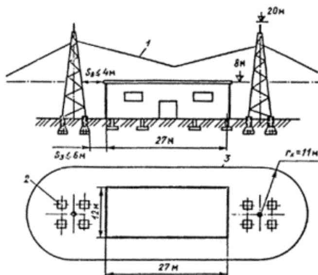
Рисунок 8 - Молниезащита здания I категории отдельно стоящим двойным стержневым молниеотводом ( \rho = 300 \text{ Ом м} , S_2 \leq 4 \text{ м} , S_3 \leq 6 \text{ м} ):
