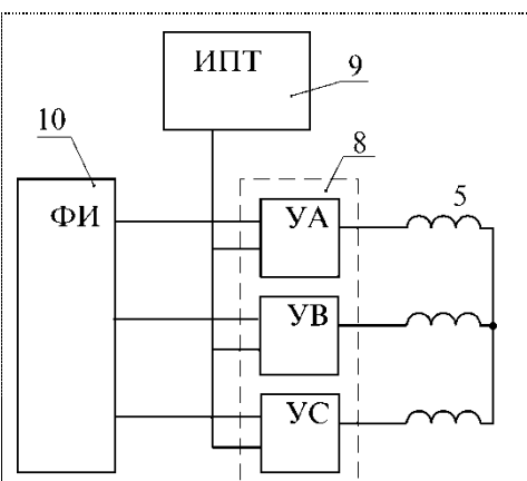
Рисунок – Функциональная схема подключения устройства.
