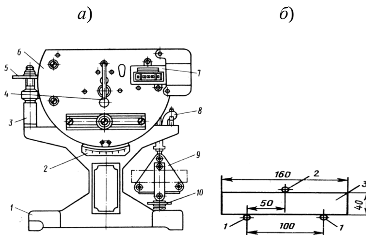
Рисунок 5.13 – Прибор МИИ-100
