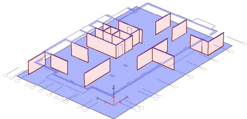
Рисунок 2.16 – Схема конструкции стен подвального этажа толщиной 200 мм
