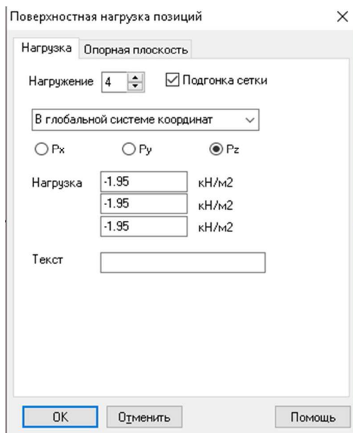
Рисунок 2.34 – Задание поверхностных нагрузок
