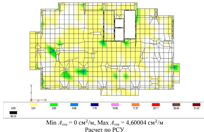
Рисунок 4.19 – Нижнее армирование вдоль локальной оси S
