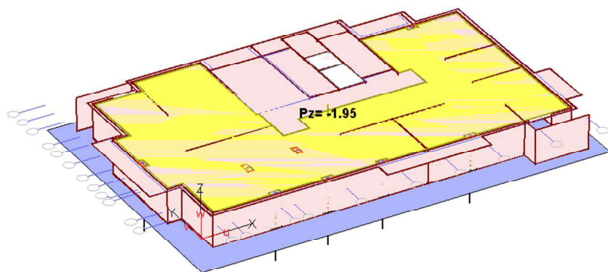
Рисунок 2.35 – Схема поверхностных нагрузок на плиту перекрытия подвального этажа в квартирах жилых зданий
