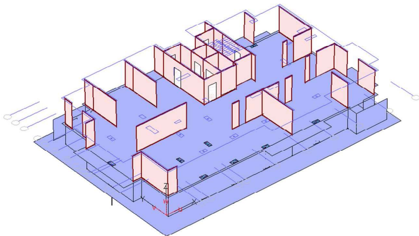
Рисунок 2.41 – Схема установленных проемов в несущих конструкциях первого этажа
