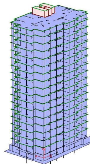
Рисунок 2.72 – Схема каркаса здания с заданными недостающими линейными опорами
