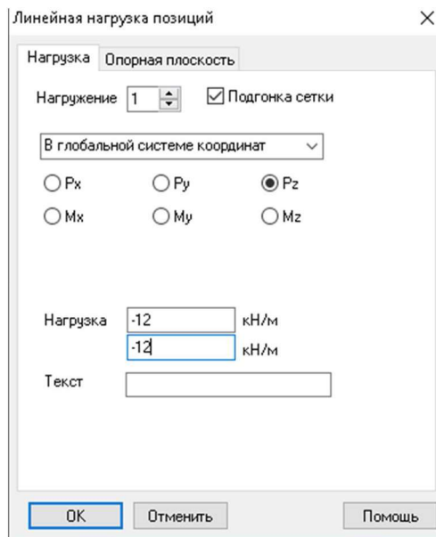
Рисунок 2.37 – Задание значений линейных нагрузок
