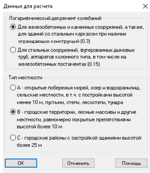
Рисунок 3.27 – Параметры логарифмического декремента колебаний и типа местности
