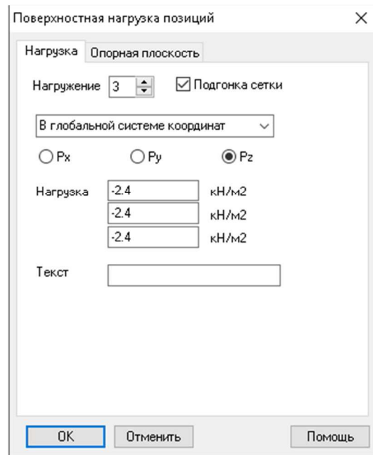
Рисунок 2.9 – Задание поверхностных нагрузок
