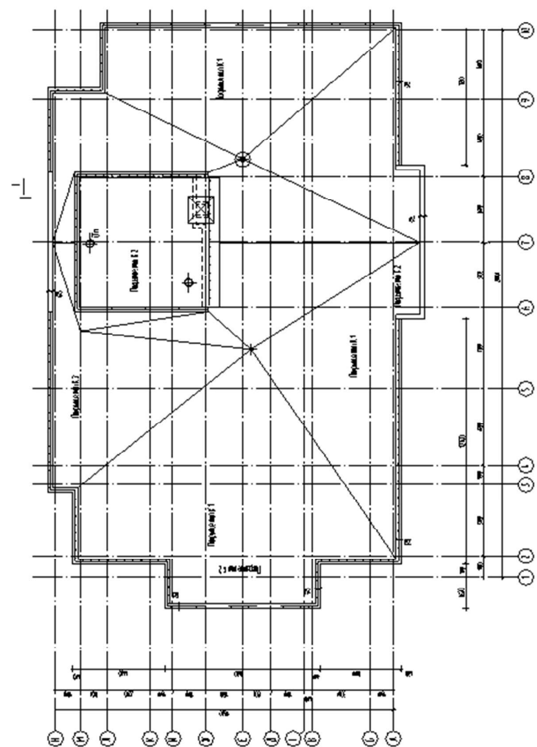
Рисунок 1.7 – План кровли
