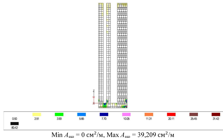
Рисунок 4.38 – Определение по расчетным сочетаниям усилий верхнего армирования вдоль локальной оси S
