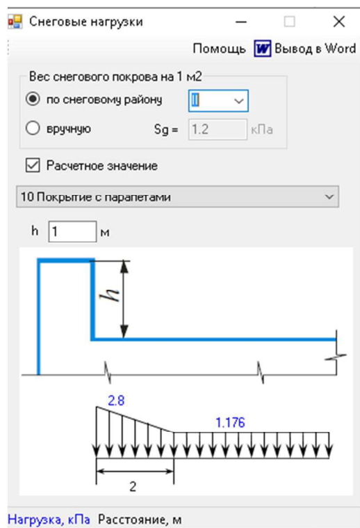
Рисунок 2.68 – Исходные данные и результаты расчета снеговой нагрузки
