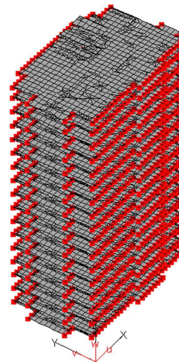
Рисунок 2.91 – Отображение выбранных узлов для генерации узловой нагрузки
