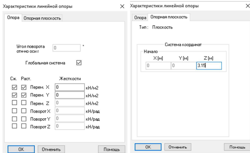
Рисунок 2.52 – Установка параметров жесткостей линейных опор
