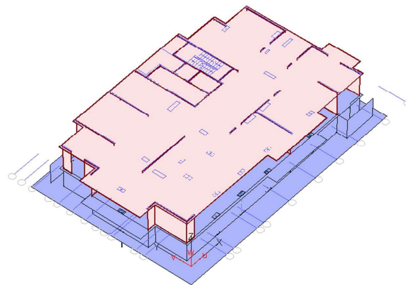
Рисунок 2.42 – Отображение установленной плиты перекрытия первого этажа
