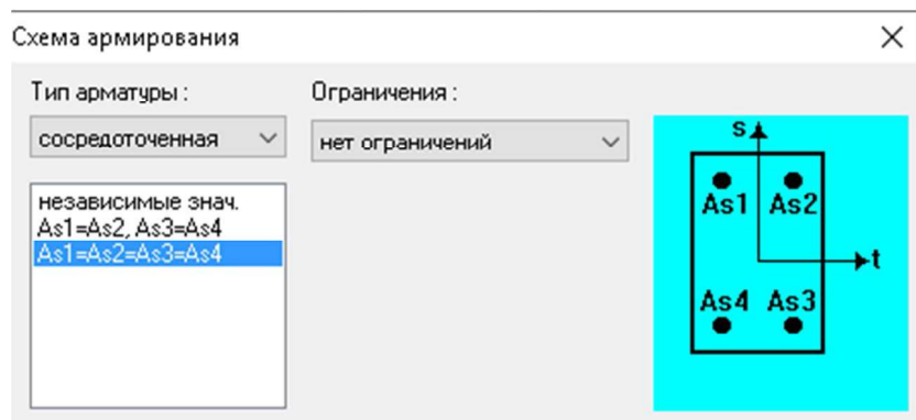
Рисунок 4.65 – Армирование рассчитываемых элементов
