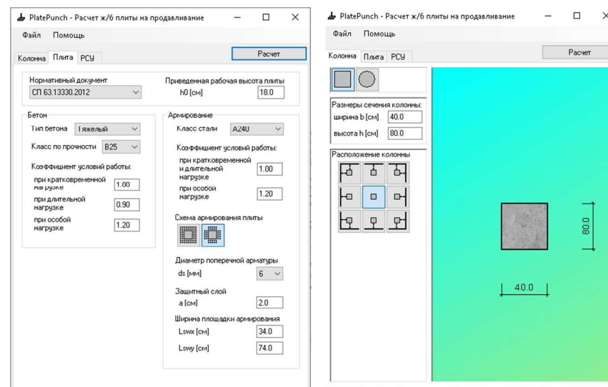
Рисунок 4.30 – Исходные данные для расчета железобетонной плиты на продавливание
