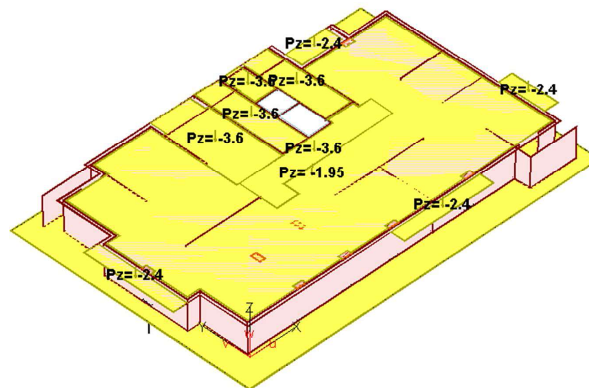
Рисунок 2.36 – Отображение поверхностных нагрузок
