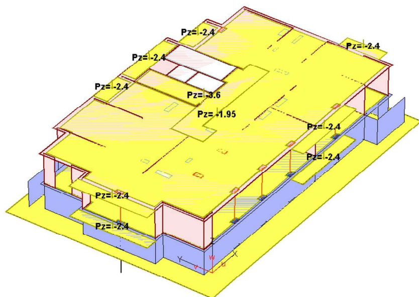
Рисунок 2.45 – Отображение всех заданных нагрузок на плиту перекрытия первого этажа
