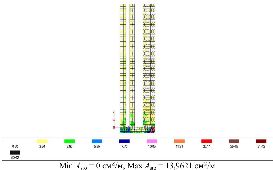
Рисунок 4.37 – Определение по расчетным сочетаниям усилий верхнего армирования вдоль локальной оси R
