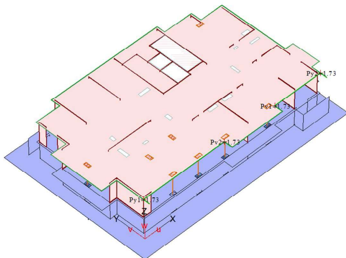
Рисунок 2.49 – Схема заданной ветровой нагрузки на наветренную сторону плиты перекрытия
