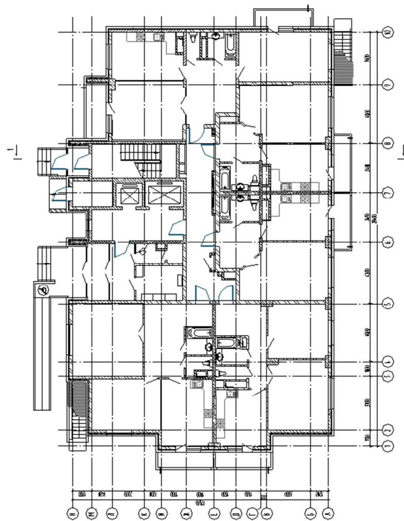
Рисунок 1.4 – План первого этажа
