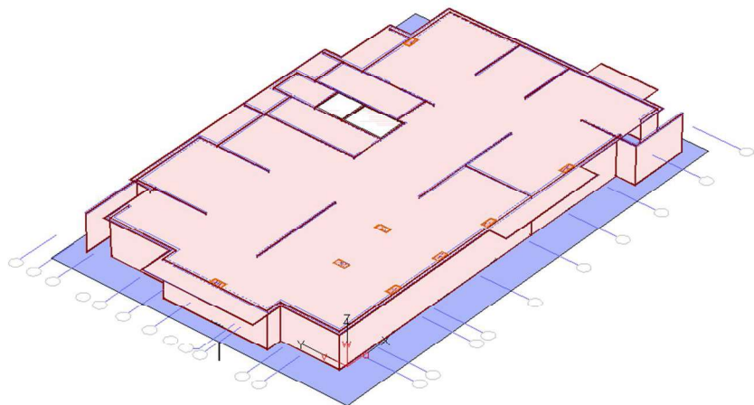
Рисунок 2.31 – Отображение установленного отверстия в плите перекрытия подвального этажа
