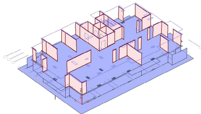
Рисунок 2.40 – Отображение вертикальных несущих конструкций первого этажа
