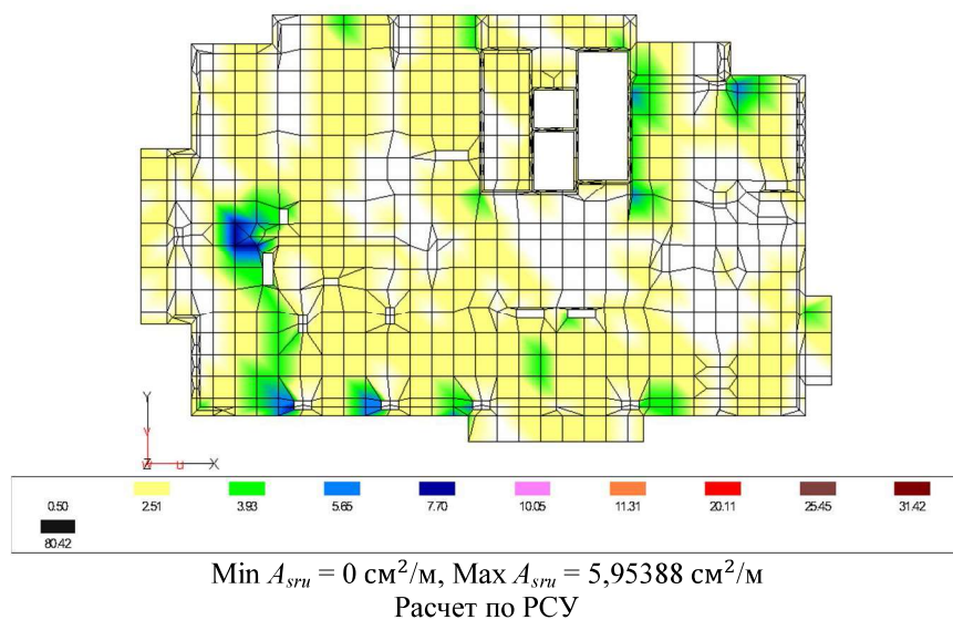
Рисунок 4.18 – Нижнее армирование вдоль локальной оси R
