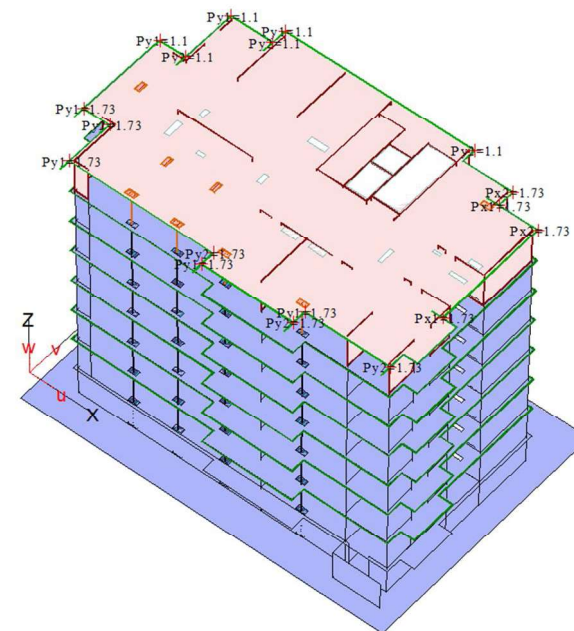
Рисунок 2.58 – Удаленная линейная нагрузка на плите перекрытия седьмого этажа
