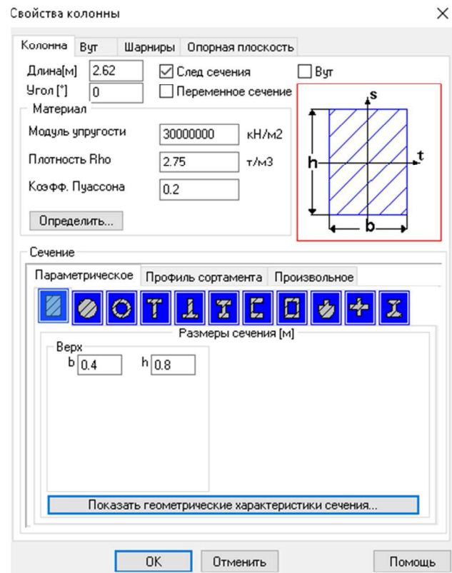
Рисунок 2.19 – Характеристики колонн подвального этажа
