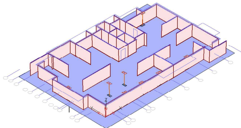
Рисунок 2.22 – Отображение конструкции колонн подвального этажа
