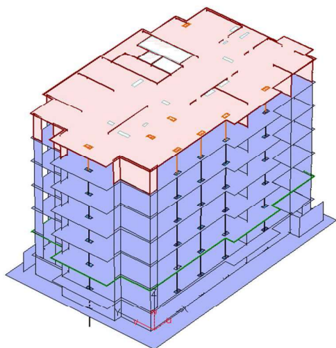
Рисунок 2.56 – Отображение каркаса здания с актуальным шестым этажом
