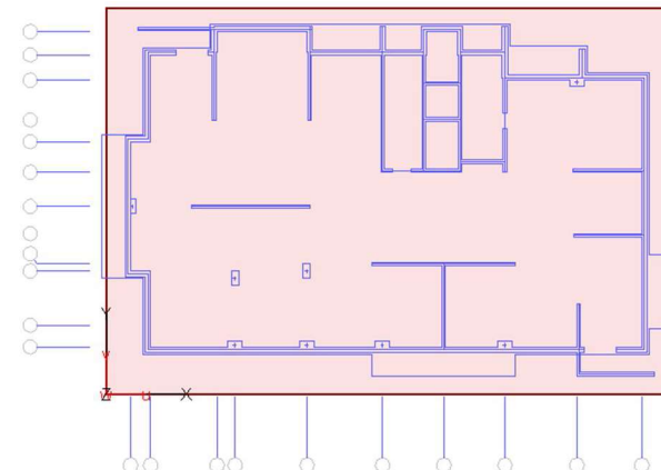
Рисунок 2.11 – Фундаментная плита с DXF подосновой конструкций подвального этажа
