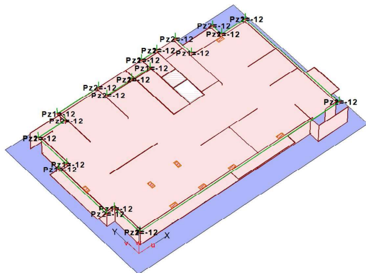
Рисунок 2.38 – Отображение линейной нагрузки на плите перекрытия подвального этажа
