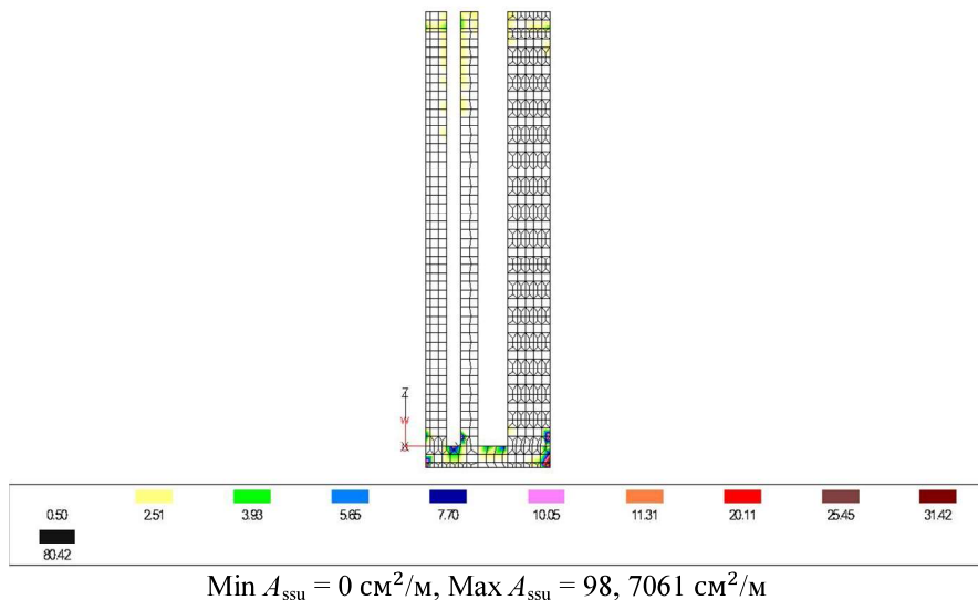
Рисунок 4.40 – Определение по расчетным сочетаниям усилий нижнего армирования вдоль локальной оси S
