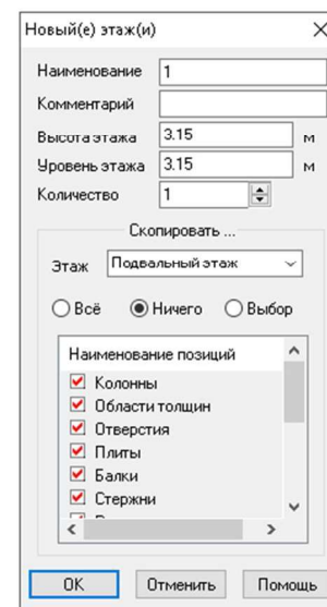
Рисунок 2.39 – Параметры вертикальных несущих конструкций первого этажа
