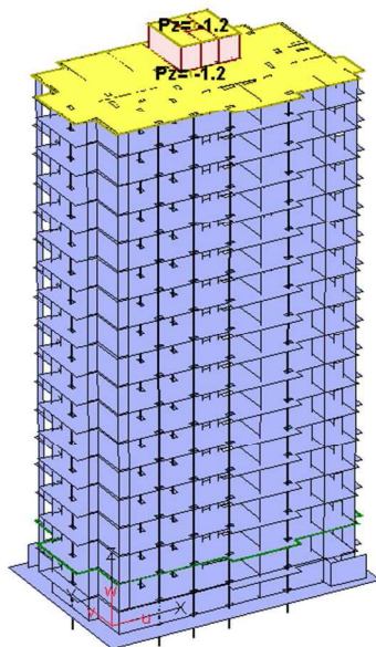
Рисунок 2.71 – Отображение каркаса с заданной снеговой нагрузкой
