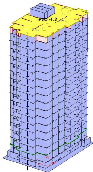
Рисунок 2.70 – Отображение каркаса с заданной снеговой нагрузкой на плиту покрытия технического этажа
