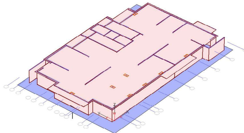
Рисунок 2.30 – Вид установленной плиты перекрытия подвального этажа
