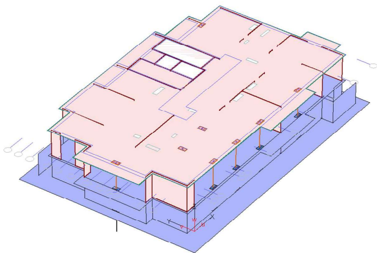
Рисунок 2.53 – Установленные линейные опоры по периметру перекрытия первого этажа
