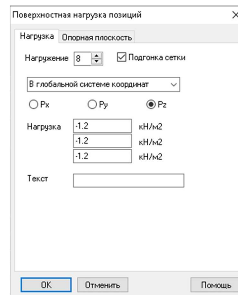
Рисунок 2.69 – Задание поверхностных нагрузок
