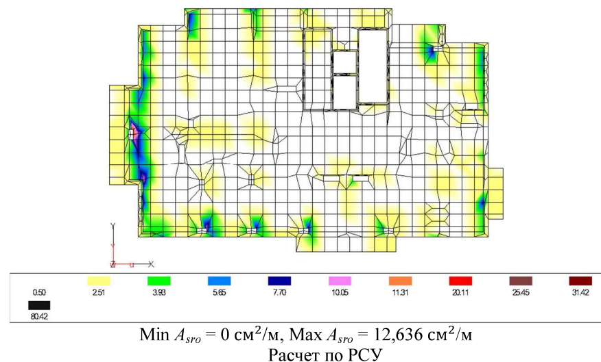
Рисунок 4.16 – Верхнее армирование вдоль локальной оси R
