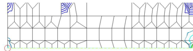
Рисунок 4.42– Выбор сечения для осреднения значений площади поперечного сечения нижнего армирования
