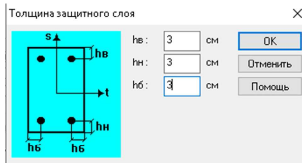
Рисунок 4.66 – Задание толщины защитного слоя рассчитываемых элементов
