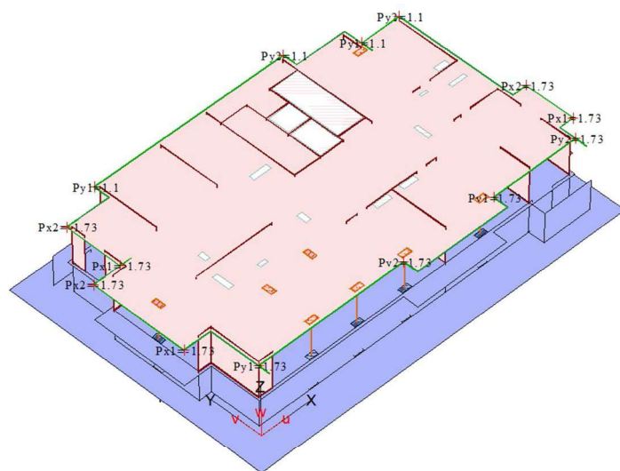
Рисунок 2.50 – Числовые значения ветровой нагрузки на плиту перекрытия первого этажа
