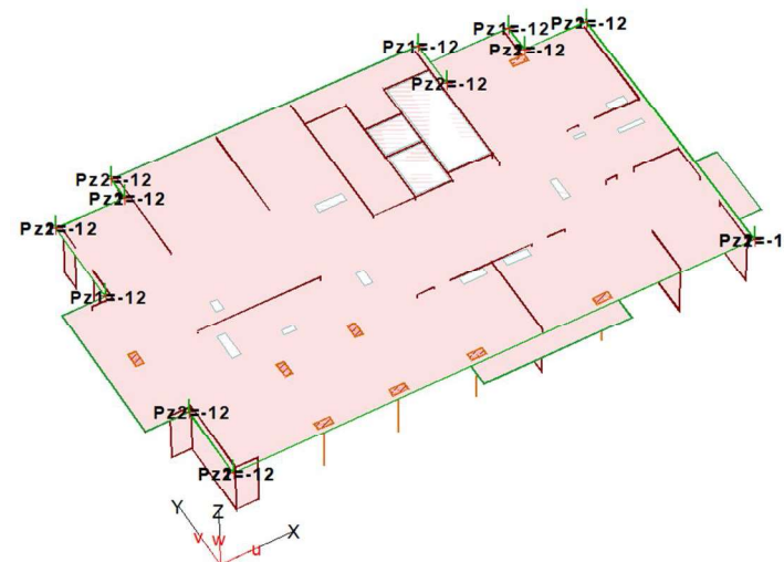
Рисунок 2.46 – Отображение всех установленных линейных нагрузок на плиту перекрытия первого этажа
