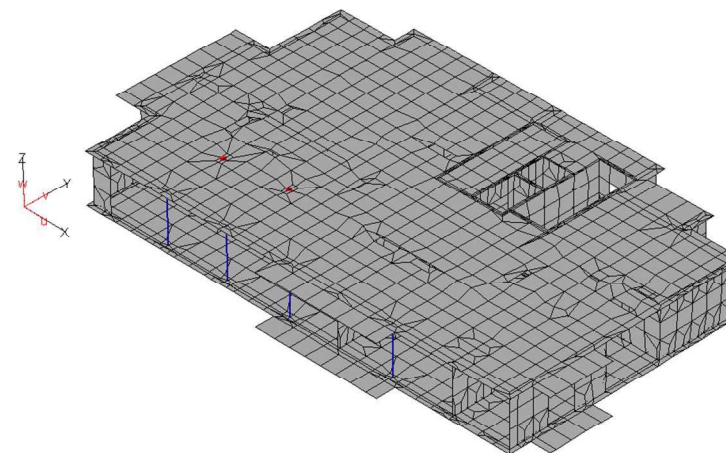
Рисунок 4.27 – Отображение рассчитываемых зон плиты перекрытия
