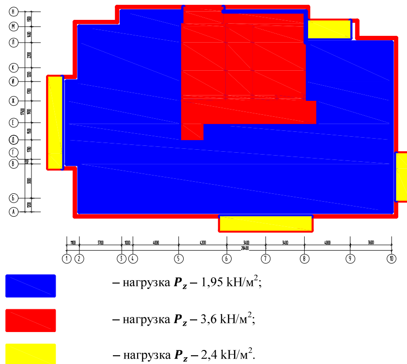
Рисунок 2.33 – Схема нагрузки на плиту перекрытия подвального этажа
