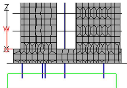
Рисунок 2.80 – Удаление фиктивных элементов
