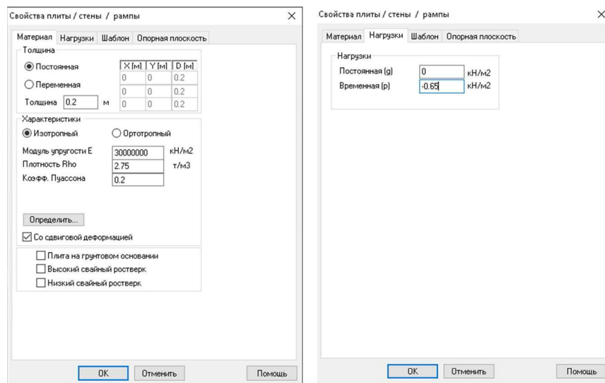
Рисунок 2.29 – Характеристики плиты перекрытия подвального этажа
