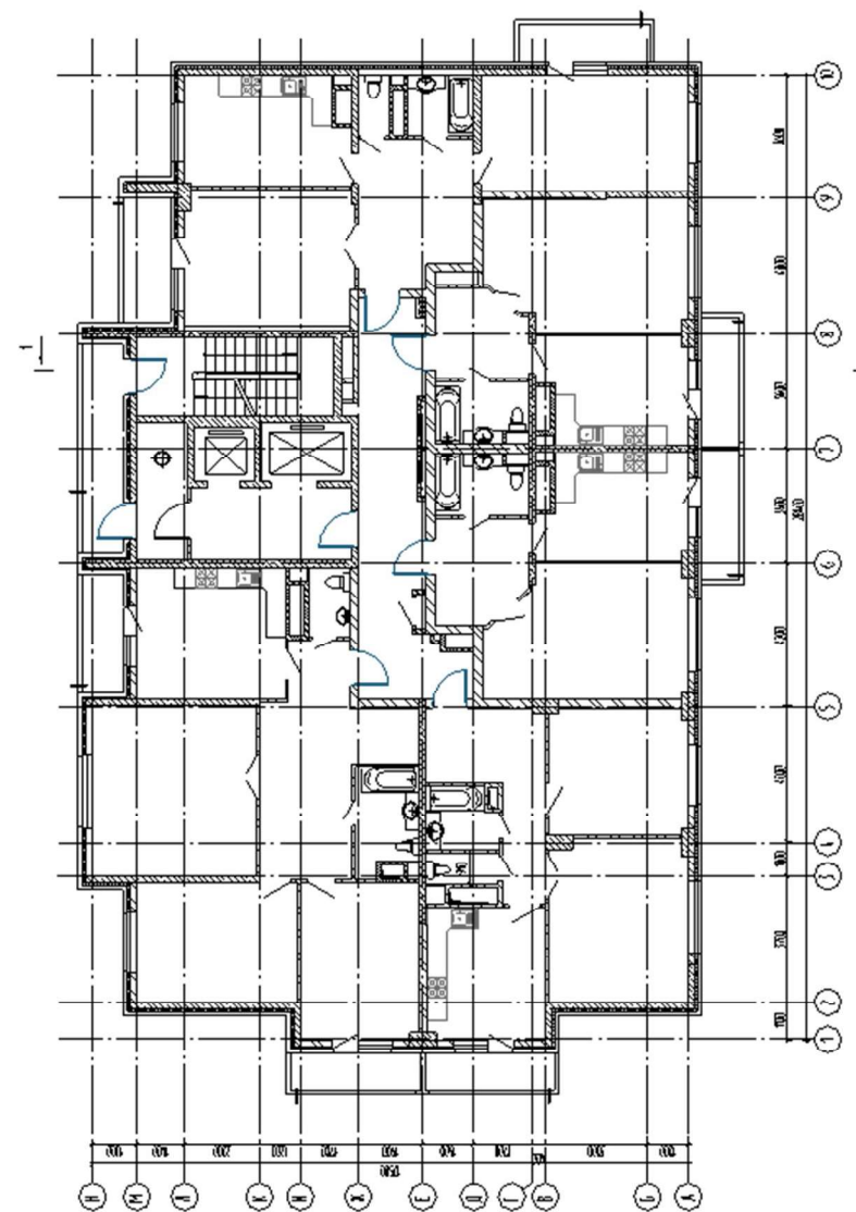
Рисунок 1.5 – План типового этажа
