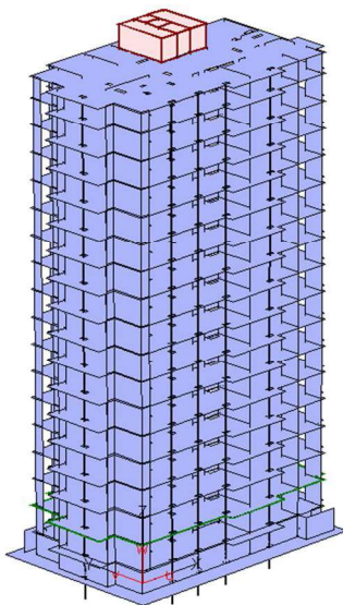
Рисунок 2.65 – Отображение каркаса здания с актуальным этажом – машинным отделением
