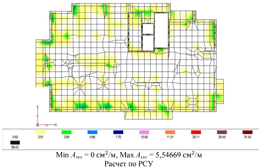
Рисунок 4.17 – Верхнее армирование вдоль локальной оси S
