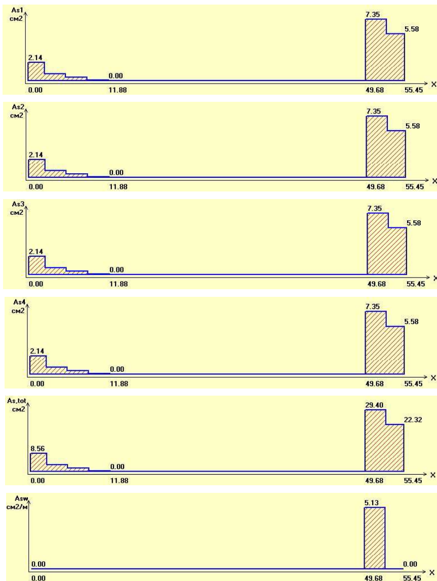
Рисунок 4.75 – Эпюры армирования стержней
