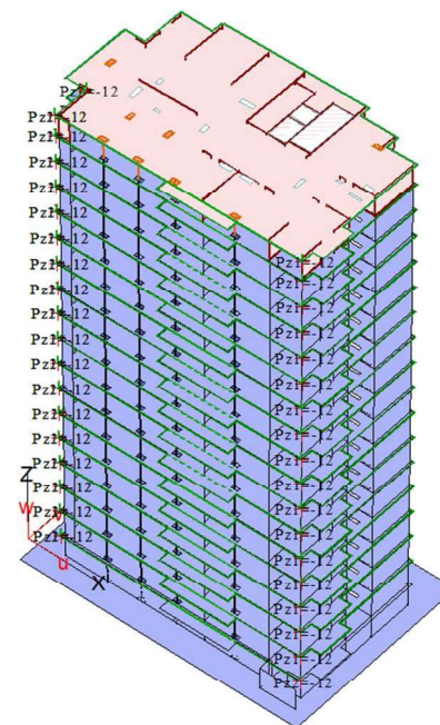
Рисунок 2.63 – Заданная ветровая нагрузка с первого по шестнадцатый и технический этаж
