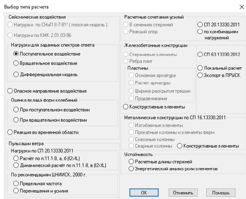
Рисунок 3.15 – Исходные данные к расчету сейсмических нагрузок
