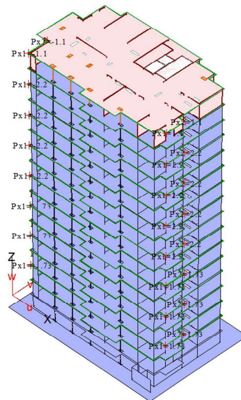
Рисунок 2.60 – Заданная ветровая нагрузка на перекрытиях с первого по шестнадцатый этаж
