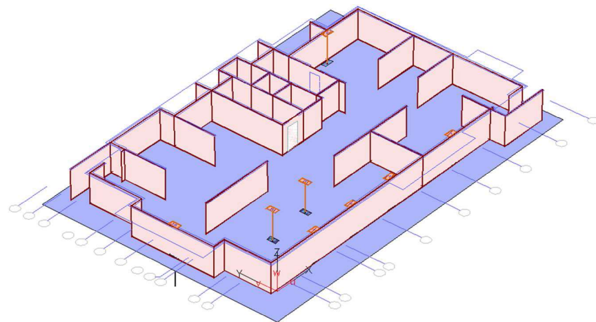
Рисунок 2.26 – Проекция установленного проема в подвальном этаже
