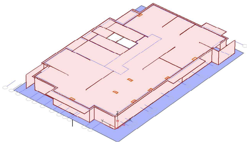
Рисунок 2.32 – Плита перекрытия подвального этажа с DXF подосновой (первый этаж нагрузки)
