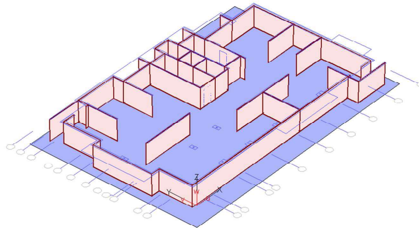
Рисунок 2.17 – Отображение конструкции стен подвального этажа
