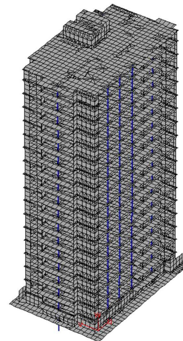
Рисунок 2.78 – Отображение сгенерированной конечно-элементной сетки
