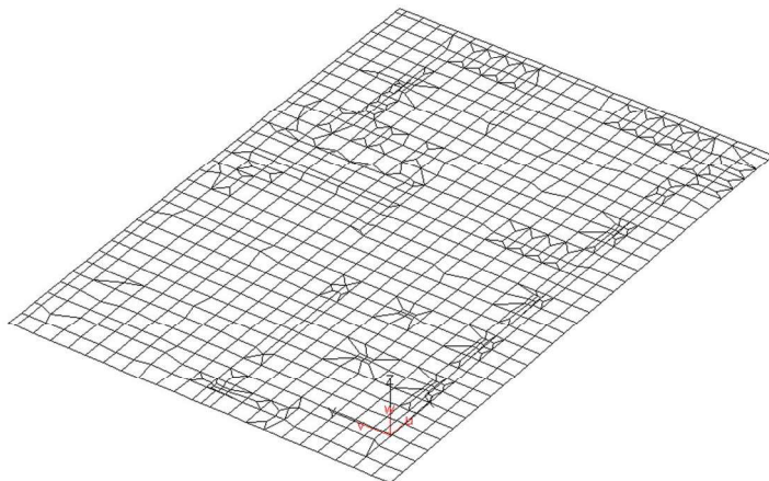
Рисунок 2.81 – Выбранный фрагмент фундаментной плиты
