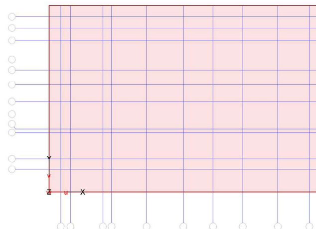
Рисунок 2.8 – Фундаментная плита
