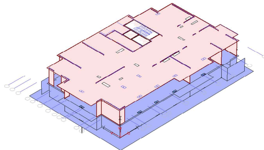
Рисунок 2.43 – Схема установленных проемов в плите перекрытия первого этажа
