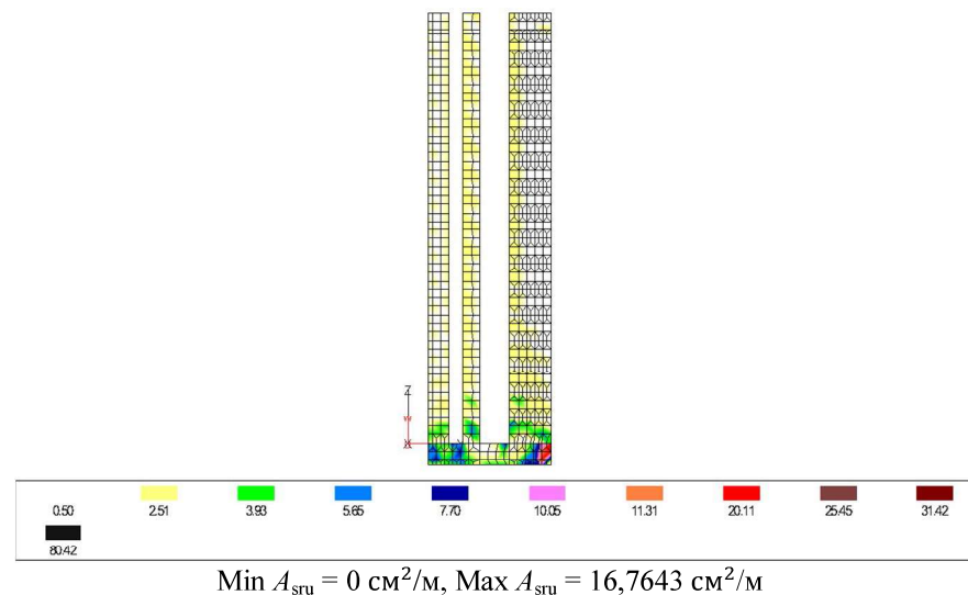
Рисунок 4.39 – Определение по расчетным сочетаниям усилий нижнего армирования вдоль локальной оси R
