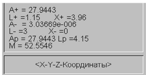
Рисунок 4.46 – Информация по эпюре распределения арматуры
