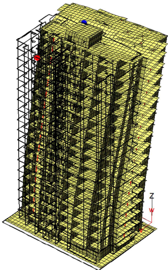
Рисунок 3.3 – Отображение первой формы собственных колебаний
