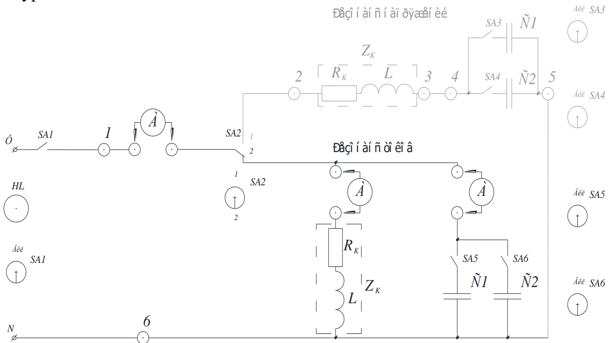
Рисунок 4.2 – Исследуемая схема
