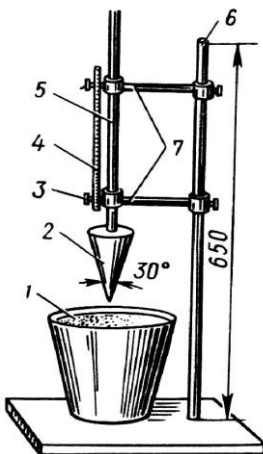
Рисунок 2.1 – Прибор для определения подвижности смеси:
