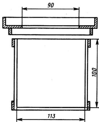
Рисунок 2.2 – Стальной цилиндрический сосуд
