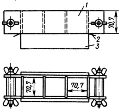
Рисунок 2.3 – Металлическая форма с поддоном
