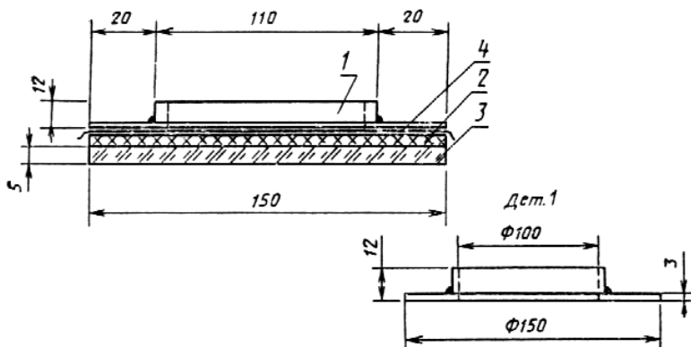
Рисунок 2.5 – Схема прибора для определения водоудерживающей способности растворной смеси
