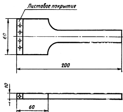
Рисунок 2.4 – Шпатель для уплотнения растворной смеси
