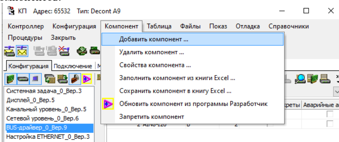
Рисунок 36 – Меню «Компонент».
