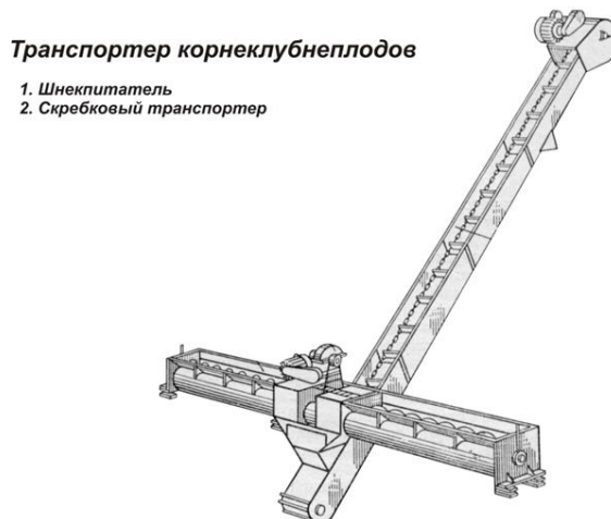
Рисунок 1 – Транспортер корнеклубнеплодов
