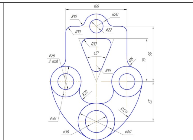
Рисунок 4 Вариант 4 Подвеска
