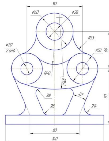
Рисунок 2 Вариант 2 Подвеска
