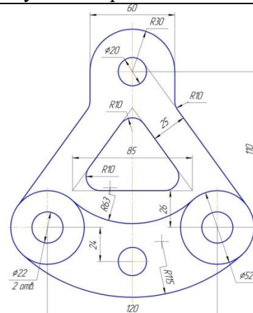
Рисунок 6 Вариант 6 Подвеска
