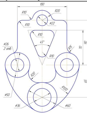
Рисунок 4 Вариант 4 Подвеска
