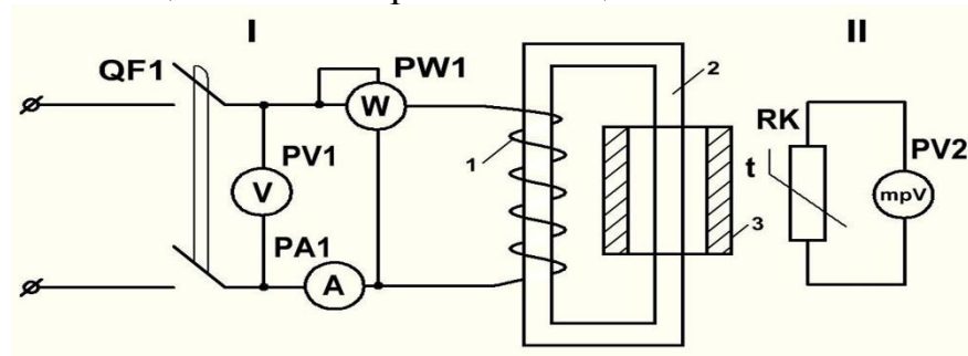
Рис. 1. Схема установки
