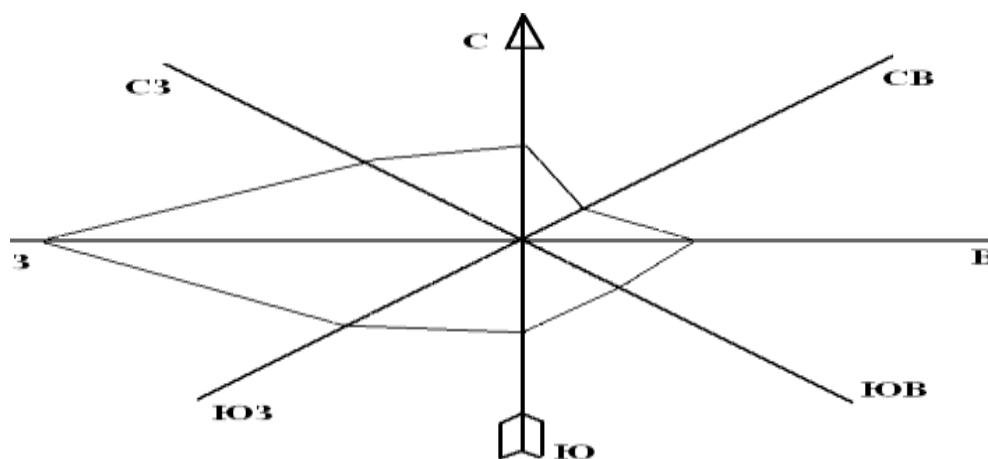
Рис. 2. Роза ветров
