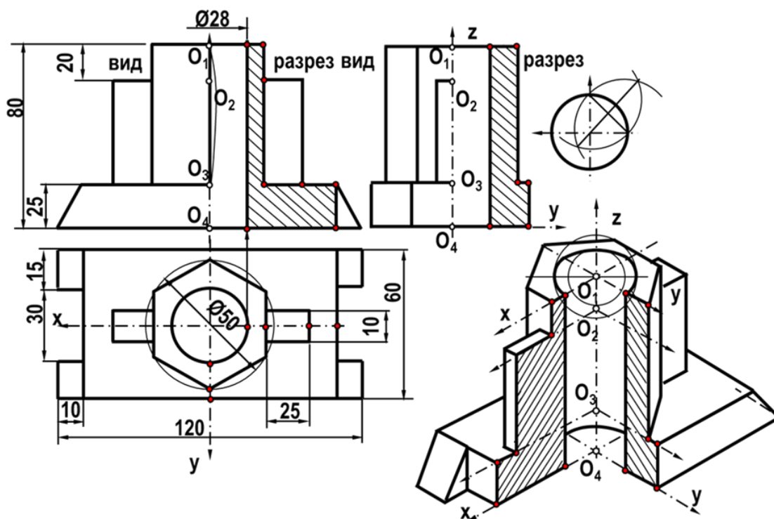
Разрезы простые
