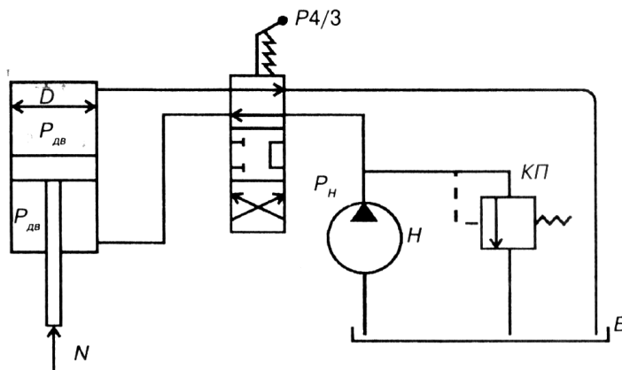
Рисунок 1 – Схема объемного гидропривода возвратно-поступательного движения
