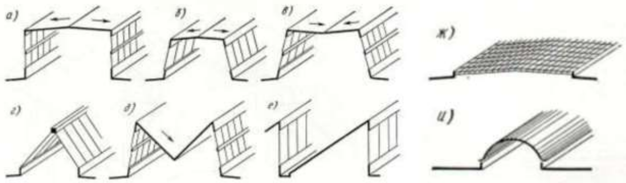
Рисунок 40 - Основные профили световых и комбинированных фонарей: а) прямоугольный; б, в) трапециевидный; г) треугольный; д) М-образный; е) шедовый; ж, и) зенитный
