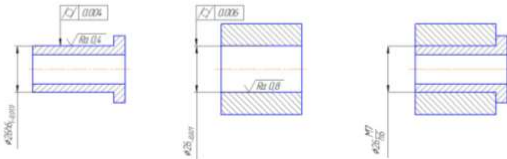
Рисунок 1.3 – Эскиз соединения посадки \varnothing 26 \begin{matrix} M7 \\ h6 \end{matrix}
