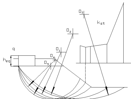
Рисунок 1 – Определение наиболее вероятной поверхности скольжения из условия минимального значения коэффициента устойчивости
