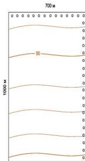
Сплошные горизонтали проведены через 2 м М 1:25000
