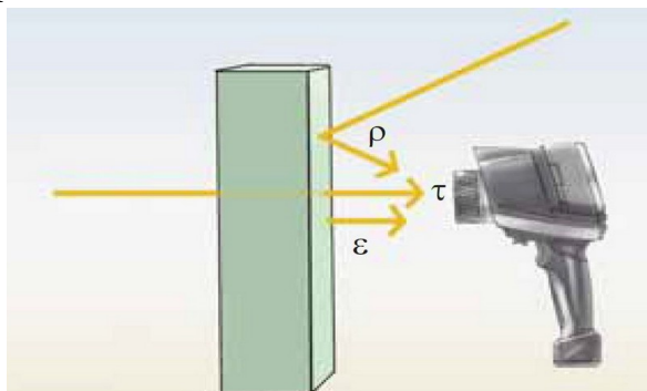
Рисунок 1.1 – К определению коэффициентов излучения, отражения и пропускания
