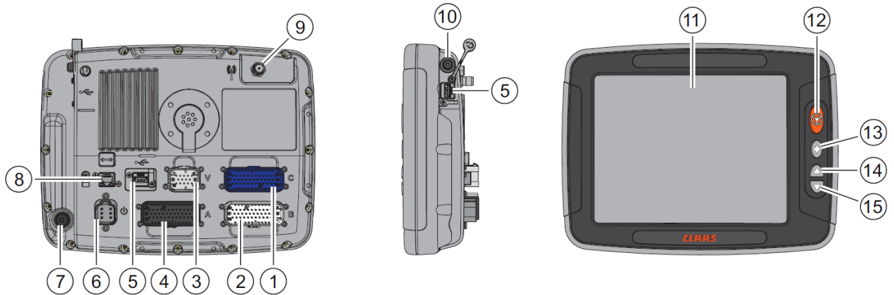
Рисунок 4 – Устройство терминала GPS PILOT S10:
