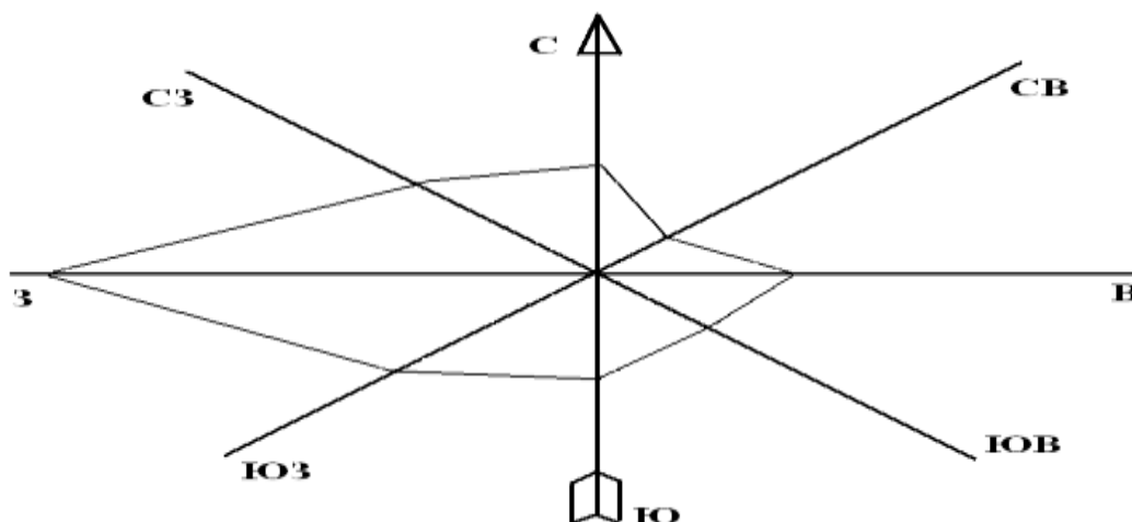
Рис. 2. Роза ветров
