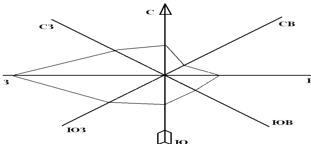
Рис. 2. Роза ветров
