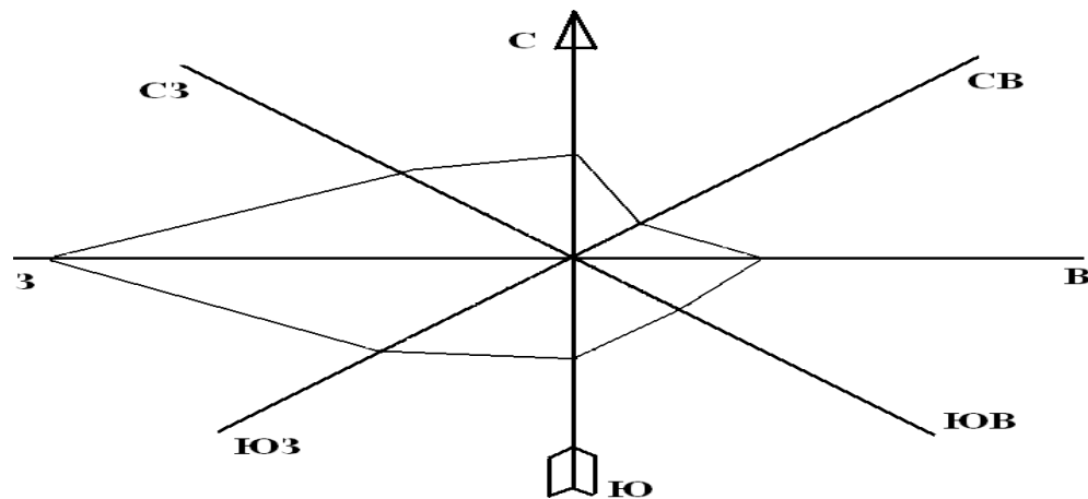
Рис. 2. Роза ветров
