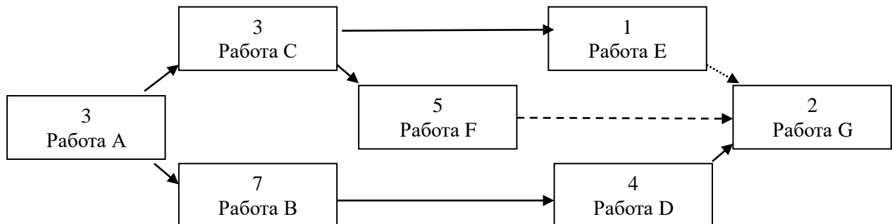
Рис. 1. Сетевая диаграмма проекта
